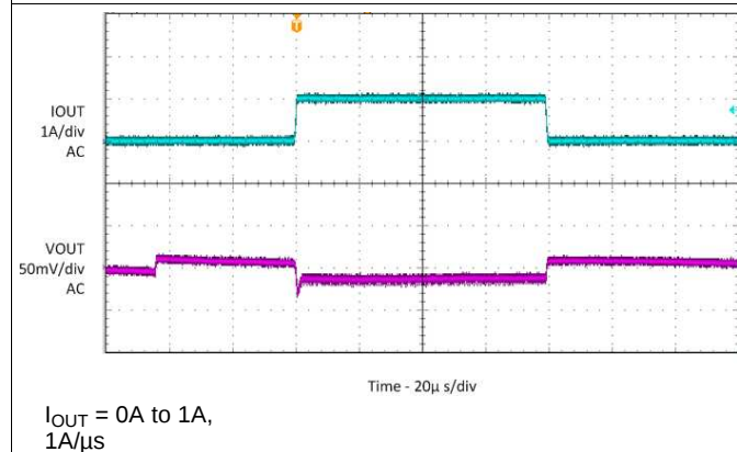
图 26. Load Transient
