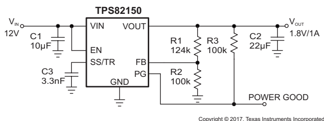
代表的なアプリケーションの回路図
