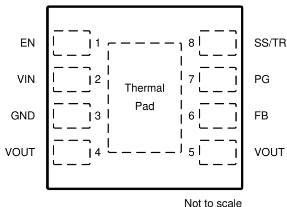
图 5-1. SIL 8-Pin µSiL Package (SIL0008C Top View)
