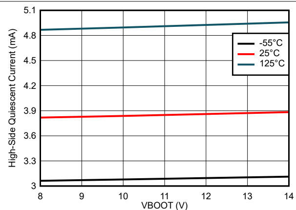
図 7-41. ハイスайд静止電流とブート電圧との関係
