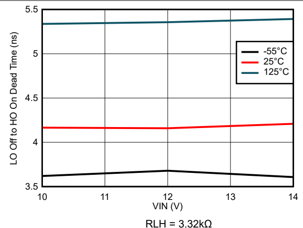
図 7-30. LO オフから HO オンのデッドタイムと VIN 電圧との関係
