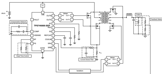
TPS7H5005-SEP の代表的なアプリケーション
