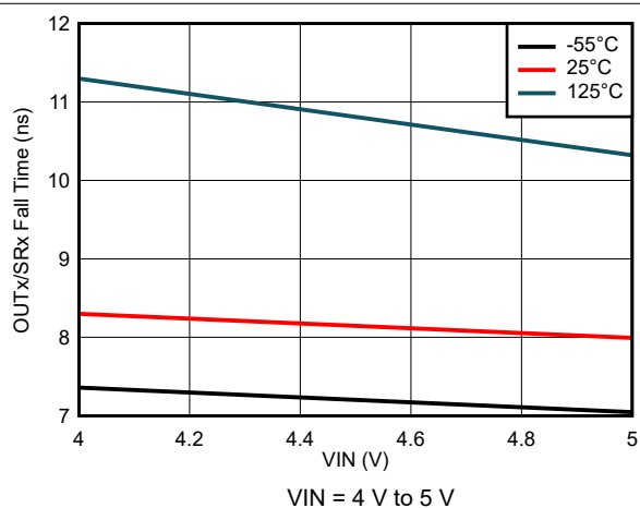
図 7-59. Output Fall Time Variation
