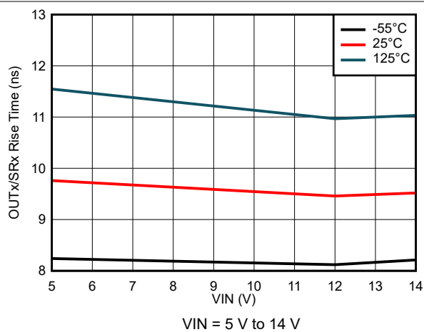
図 7-58. Output Rise Time Variation
