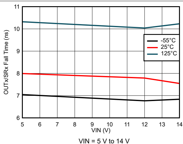
図 7-60. Output Fall Time Variation
