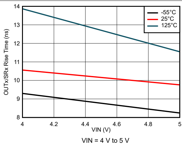
図 7-57. Output Rise Time Variation
