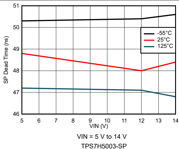
図 7-56. SP Dead Time Variation
