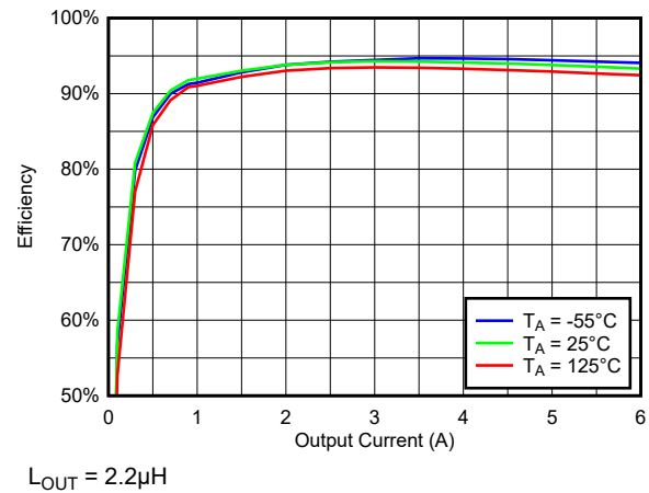
図 7-16. 温度全体に対する効率と負荷との関係 (500kHz、VIN = 12V、VOUT = 5V)
