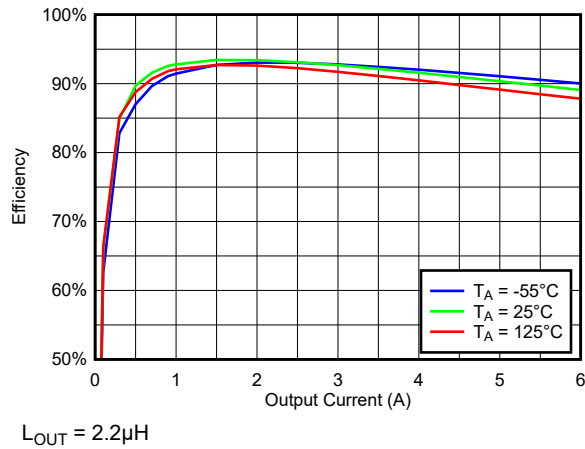
図 7-13. 温度全体に対する効率と負荷との関係 (500kHz、VIN = 5V、VOUT = 2.5V)
