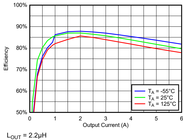
図 7-15. 温度全体に対する効率と負荷との関係 (500kHz、VIN = 5V、VOUT = 1.1V)
