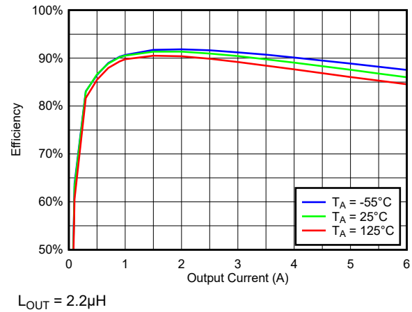
図 7-14. 温度全体に対する効率と負荷との関係 (500kHz、VIN = 5V、VOUT = 1.8V)
