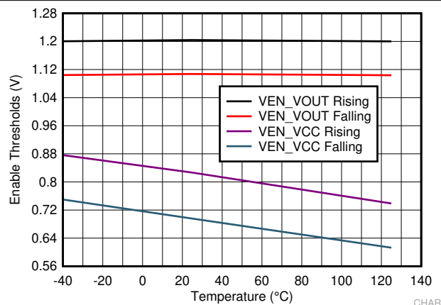
FIG 6-8. Enable Thresholds
