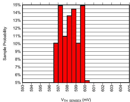
図 6-12. V_{TH\_SENSEx} 電流分布 (温度 125°C)
