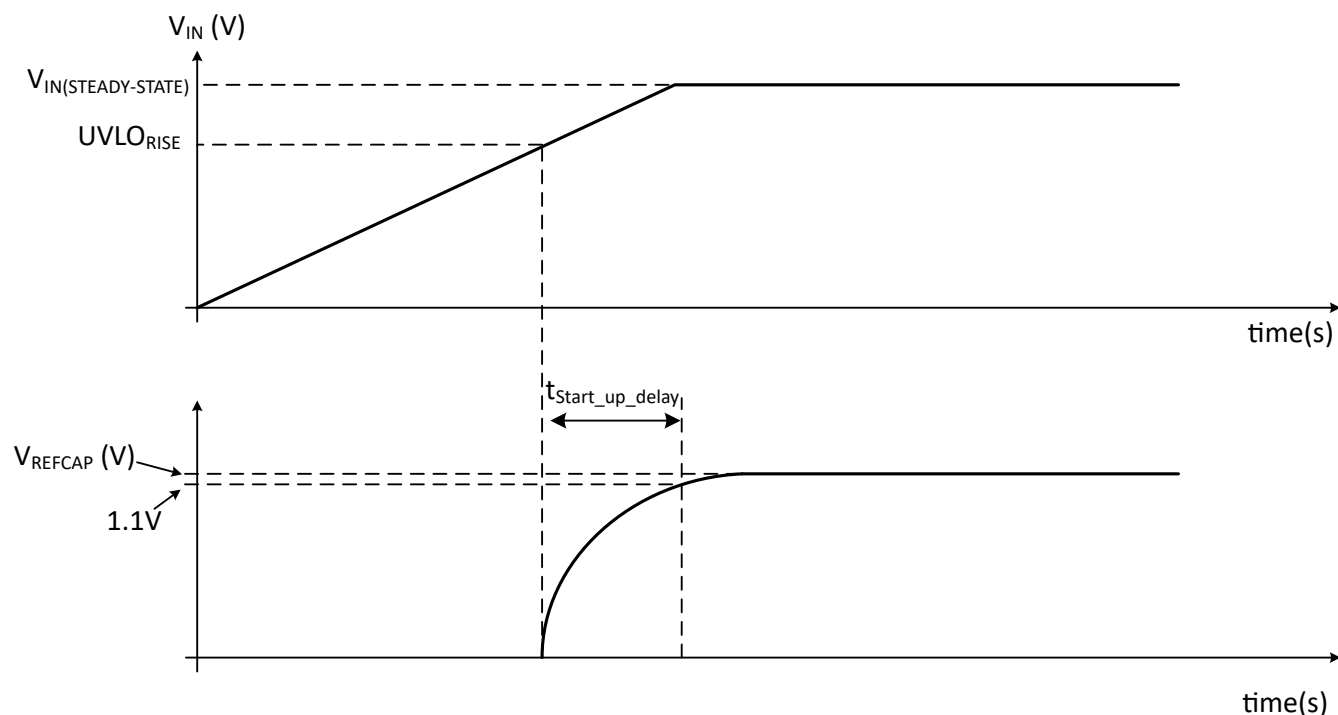
図 7-1. t_{\text{Start\_up\_delay}} 時間測定
