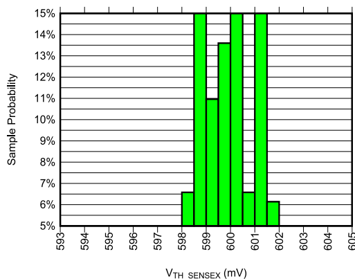
図 6-11. V_{TH\_SENSEx} 電流分布 (温度 +25°C)
