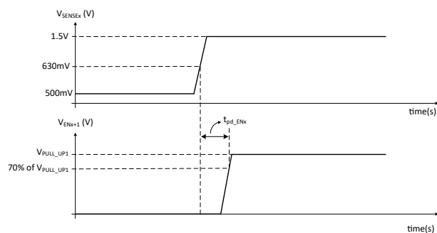
図 7-2. ENx 伝搬遅延 ( t_{\text{pd\_ENx}} ) 時間測定-立ち上がり電圧
