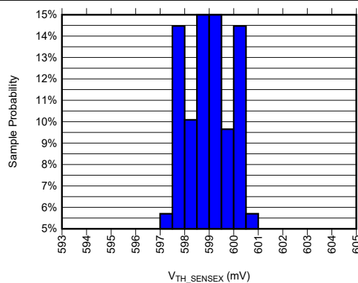
図 6-10. V_{TH\_SENSEx} 電流分布 (温度 -55°C)
