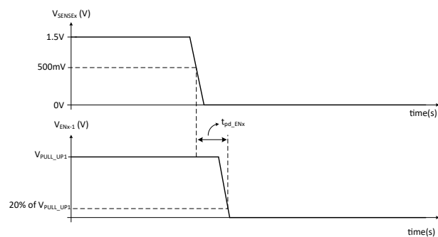
図 7-3. ENx 伝搬遅延 ( t_{\text{pd\_ENx}} ) 時間測定-立ち下がり電圧
