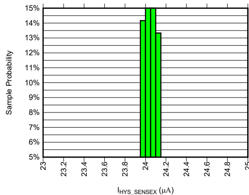
図 6-8. I_{HYS\_SENSEx} 電流分布 (温度 25°C)
