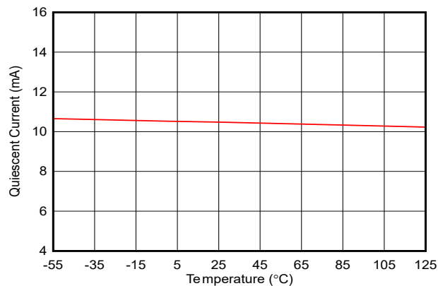
図 6-7. Quiescent Current vs Temperature
