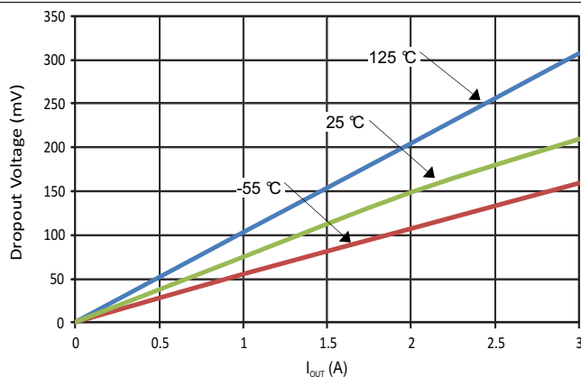
図 24. VDO vs I_{OUT}
