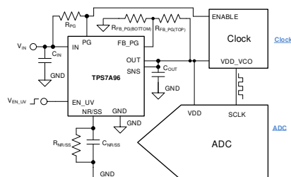
代表的なアプリケーション回路
