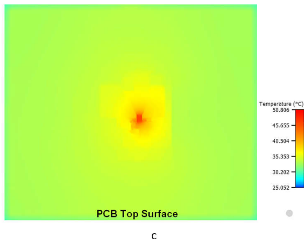
図 8-24. TPS7A96EVM-106 PCB Thermal Gradient
