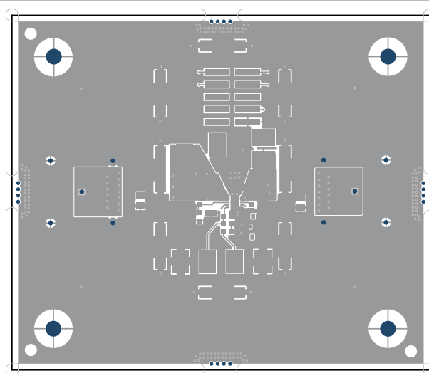
图 8-19. Top Layer Routing
