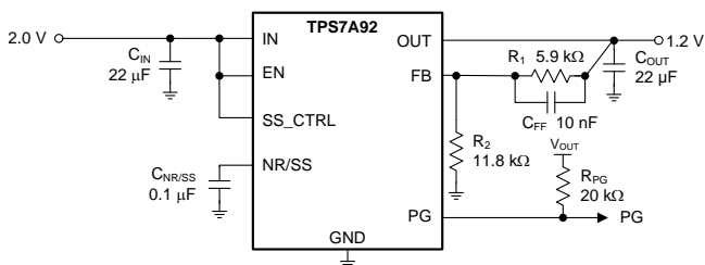
代表的なアプリケーション回路
