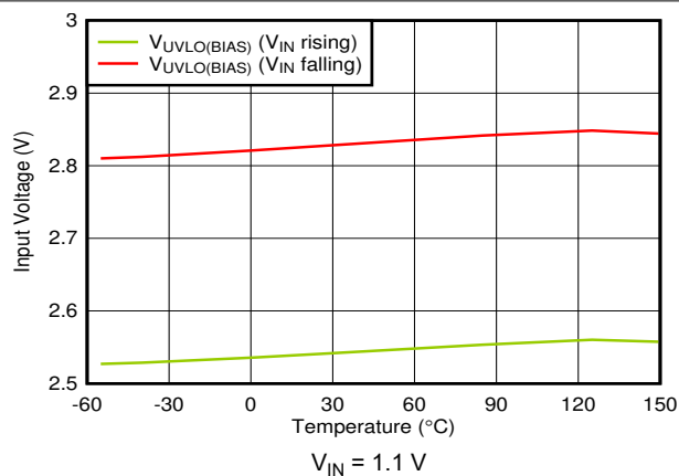
FIG 7-63. V_{BIAS} UVLO vs Temperature
