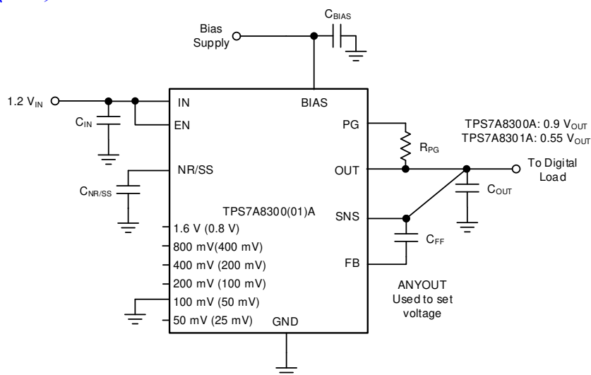
代表的なアプリケーション回路
