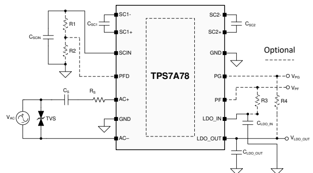
フルブリッジ構成の標準的な回路図
