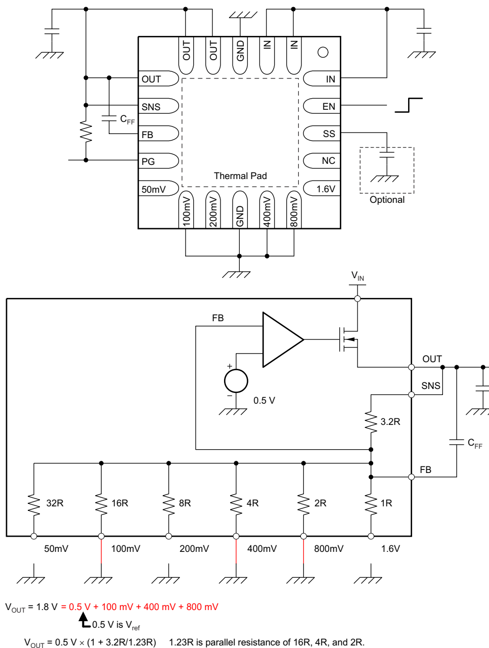
図 6-3. 1.8-V Configuration
