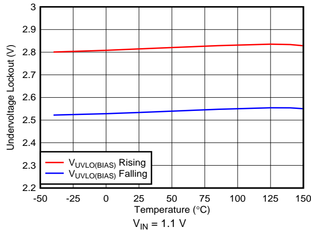
33. V_{BIAS} UVLO vs Temperature
