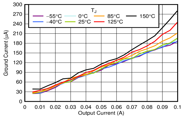
FIG 6-7. I_{\text{GND}} vs I_{\text{OUT}}
