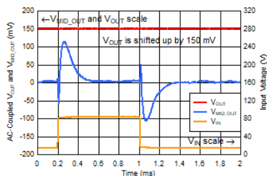
ライン過渡 ( V_{MID\_OUT} = 12V 、 V_{OUT} = 3.3V 、 I_{OUT} = 50mA )
