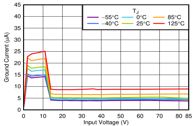
FIG 6-8. I_{\text{GND}} vs V_{\text{IN}}
