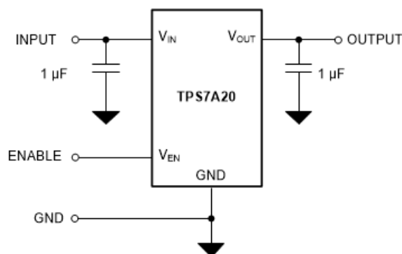
アプリケーション回路図
