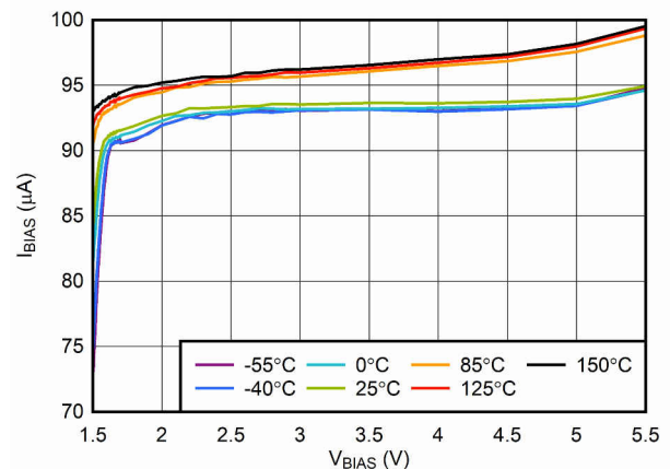
FIG 6-6. V_{\text{BIAS}} Input Current vs V_{\text{BIAS}}
