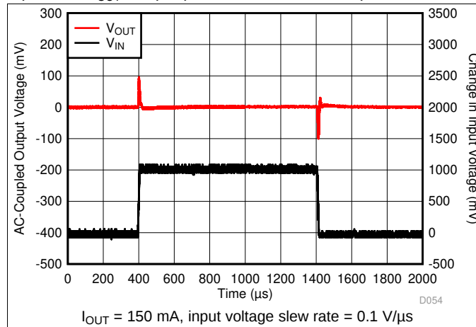
FIG 19. V_{IN} Transient
