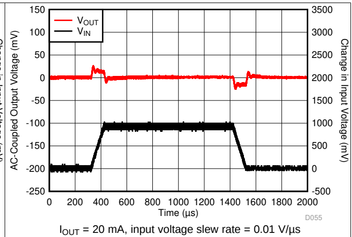
FIG 20. V_{IN} Transient
