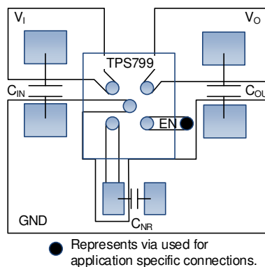
✎ 10-1. Layout Example
