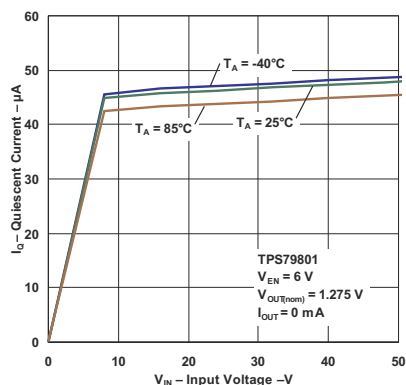
図 5-7. Quiescent Current vs Input Voltage
