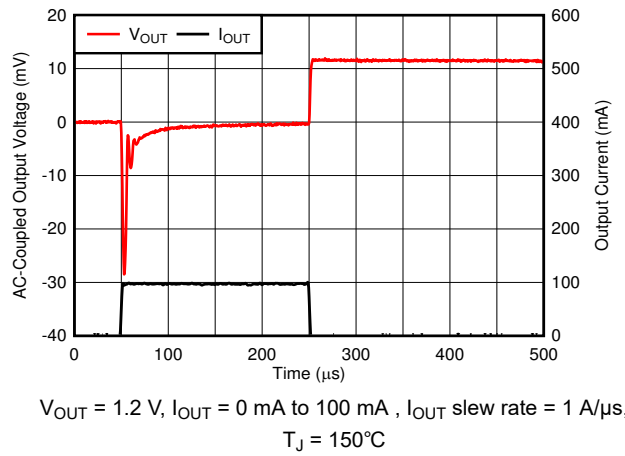
FIG 6-49. Load Transient
