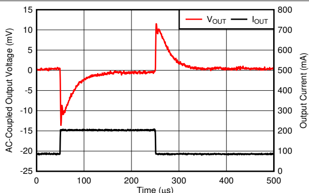
FIG 6-62. Load Transient
