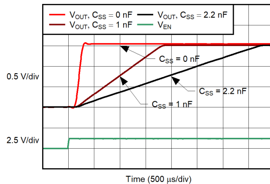
図 7-3. Turn-On Response
