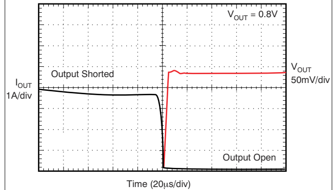
図 7-7. Output Short-Circuit Recovery
