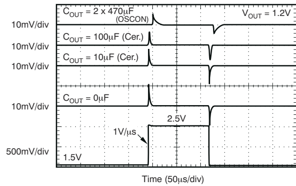
図 7-5. V_{IN} Line Transient (3A)
