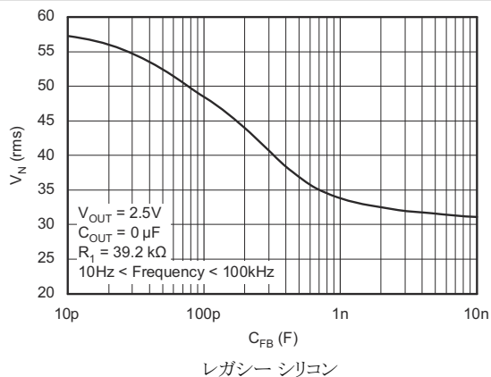
図 5-47. TPS73601 の RMS ノイズ電圧と C_F との関係
