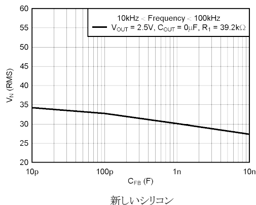
図 5-48. TPS73601 の RMS ノイズ電圧と C_F との関係
