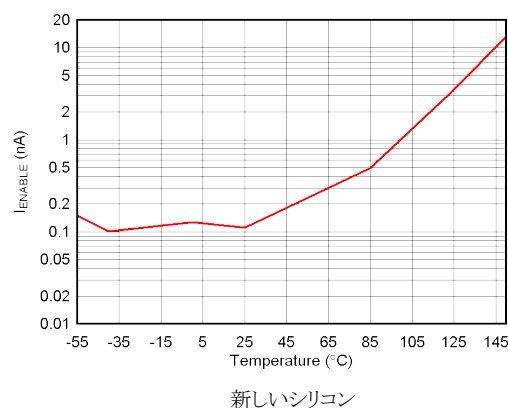
図 5-46. I_{ENABLE} VS 温度
