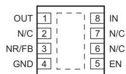
図 4-2. DRB パッケージ、8 ピン VSON (上面図)
