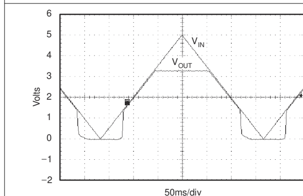
図 5-21. TPS73233 のターンオン応答
