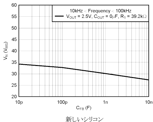
図 5-48. TPS73201 の RMS ノイズ電圧と C_{FB} との関係
