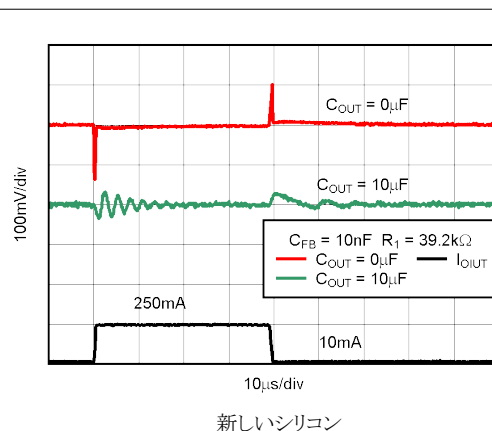
図 7-10. TPS73201 の負荷過渡応答、可変バージョン
