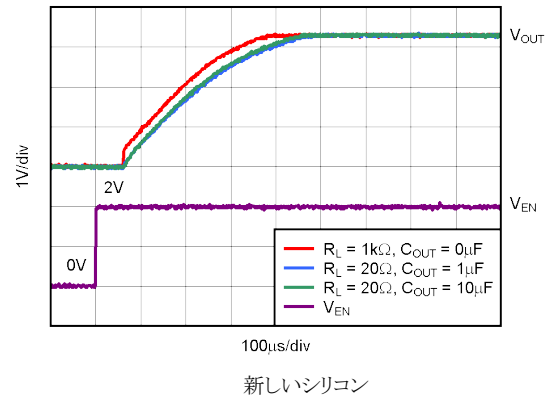
図 7-4. TPS73233 のターンオン応答
