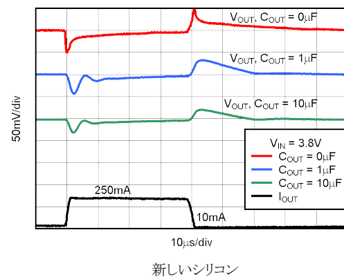
図 5-36. TPS73233 の負荷過渡応答
