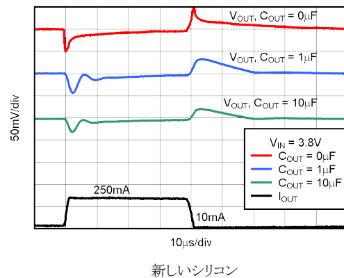
図 7-6. TPS73233 の負荷過渡応答
