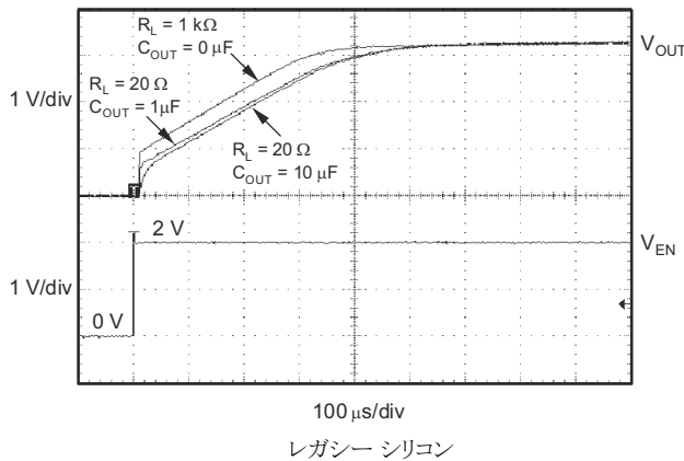
図 7-3. TPS73233 のターンオン応答
