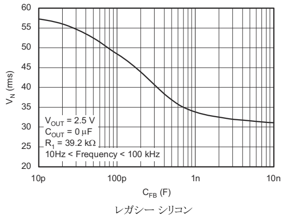
図 7-7. TPS73201 の RMS ノイズ電圧と C_{FB} との関係
