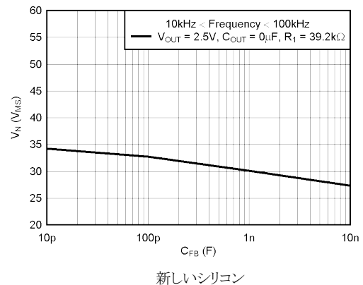
図 7-8. TPS73201 の RMS ノイズ電圧と C_{FB} との関係
