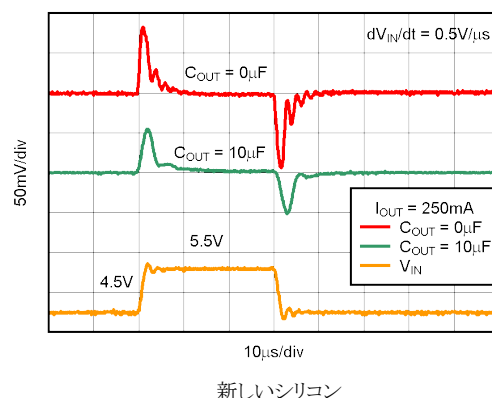
図 5-38. TPS73233 のライン過渡応答
