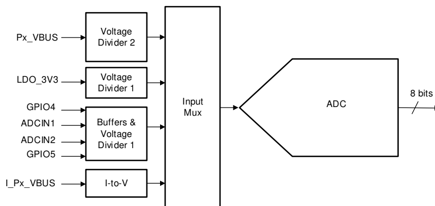
图 8-18. SAR ADC
