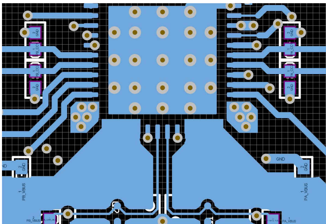
FIG 11-6. VBUS1 and VBUS2 Copper Pours and Via Placement (Top)
