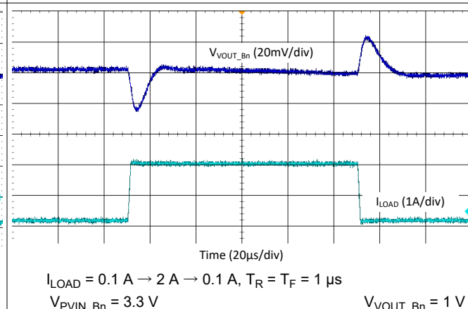
図 9-51. Buck Load Step Transient - Buck4, 4.4 MHz, Auto Mode
