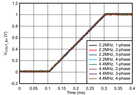
図 7-4. Buck Ramp-up Slew Rate
