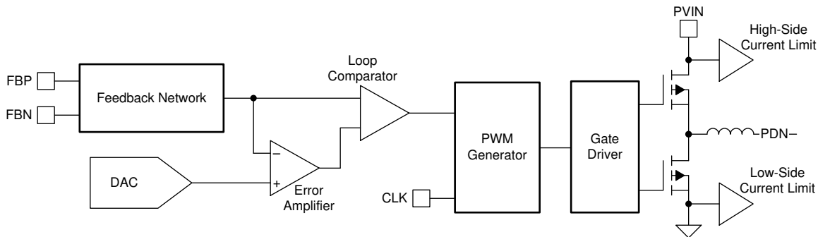
図 8-2. BUCK Core Block Diagram
