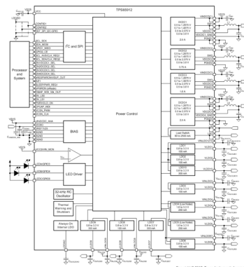
概略回路図
