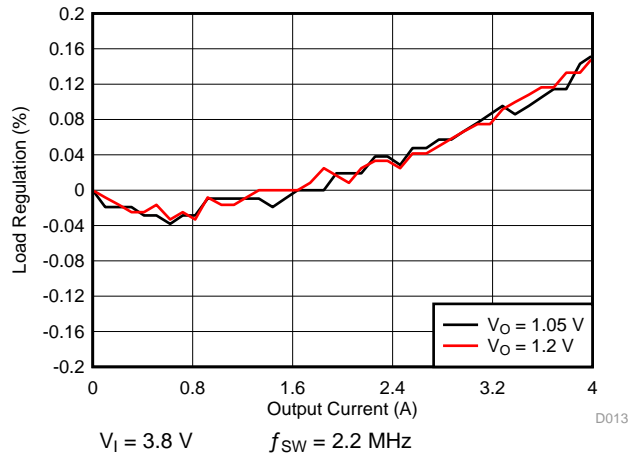
图 6-9. SMPS Load Regulation for 4-A Dual Phase
