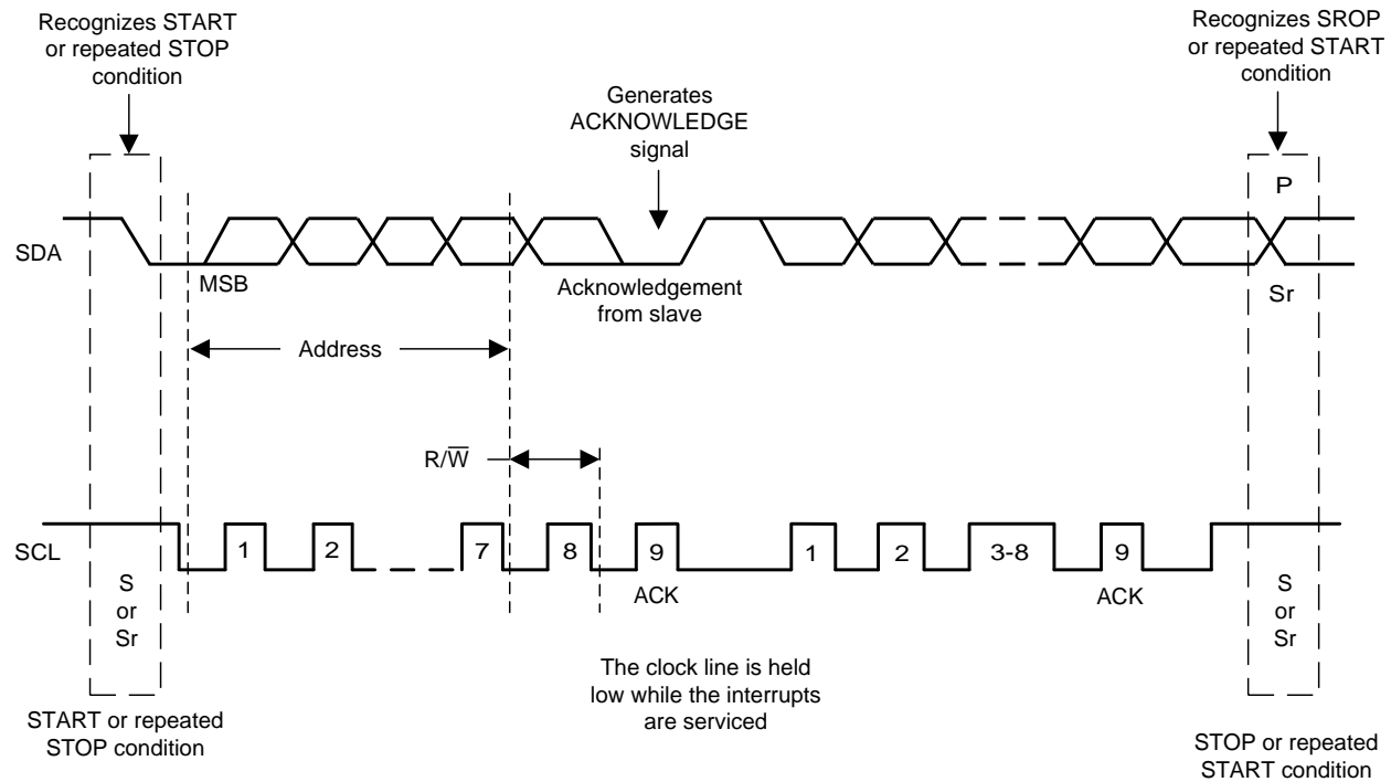
図 5-14. Bus Protocol
