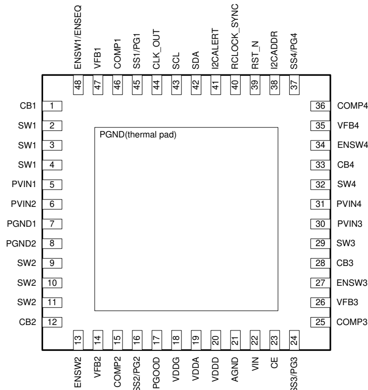
図 6-1. 48-Pin VQFN RGZ Package (Top View)
