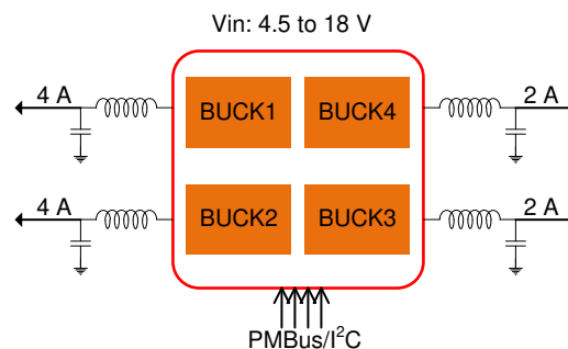
概略回路図
