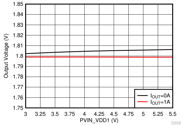
8-9. VDD1 Line Regulation, V_{OUT} = 1.8 V
