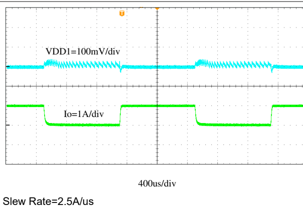
8-26. VDD1 Transient Response, 0 A to 1 A
