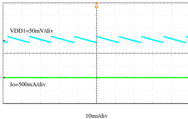
8-11. VDD1 Output Voltage Ripple, I_{OUT} = 0 A
