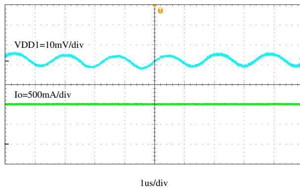
8-13. VDD1 Output Voltage Ripple, I_{OUT} = 1 A
