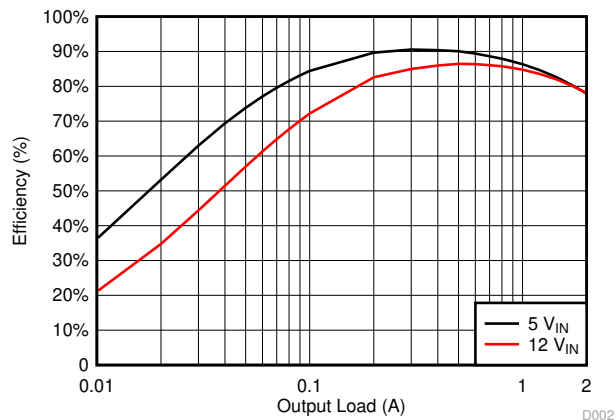
图 6-2. BUCK2 Efficiency
