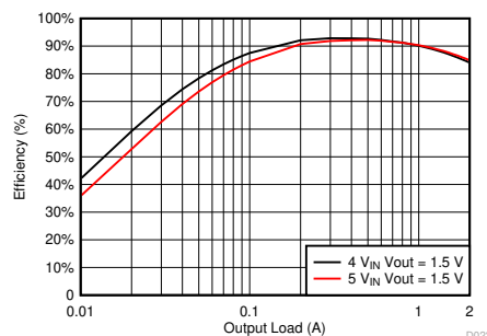
効率と出力負荷との関係
