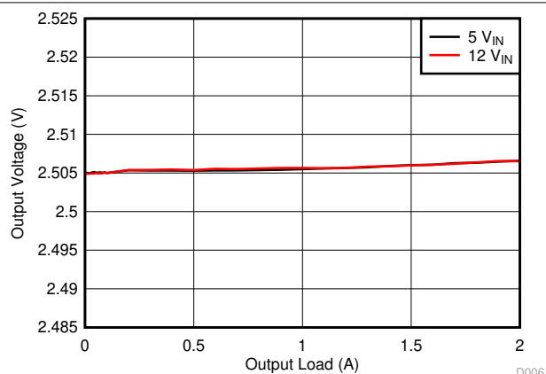
图 6-6. BUCK3, Load Regulation
