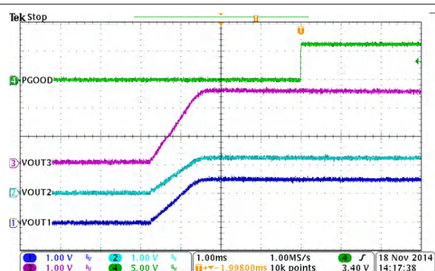
图 8-18. PGOOD
