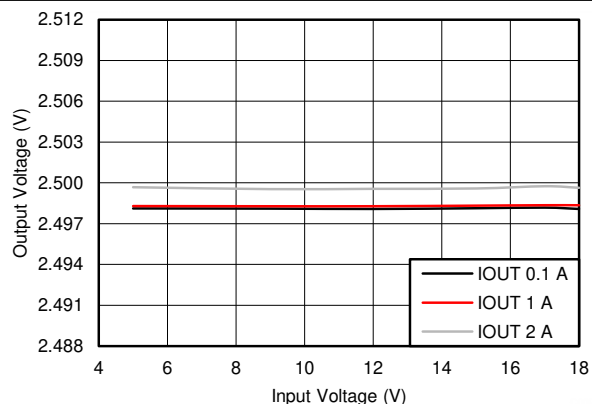
图 7-9. BUCK3, Line Regulation
