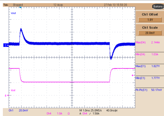
8-29. Buck 2 Dynamic Response, 1-A to 2-A Step
