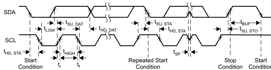
図 7-9. I 2 C Interface Timing Diagram
