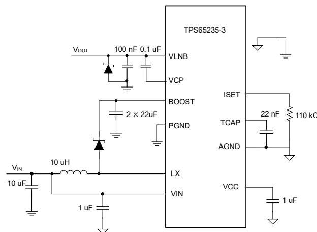
簡略回路図
