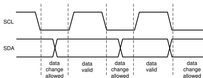
图 6-4. Data Validity Diagram
