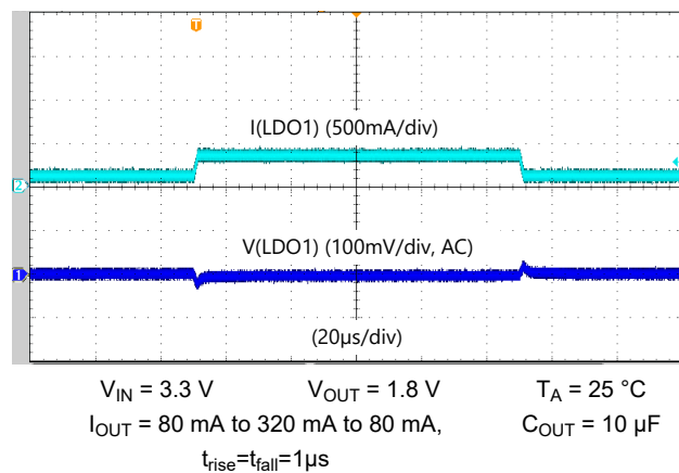
图 5-6. LDO1 Load-step response
