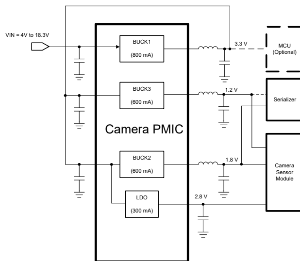
TPS650340-Q1 アプリケーション回路
