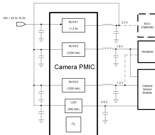
TPS650332-Q1 アプリケーション回路
