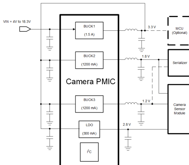
TPS650330-Q1 アプリケーション回路
