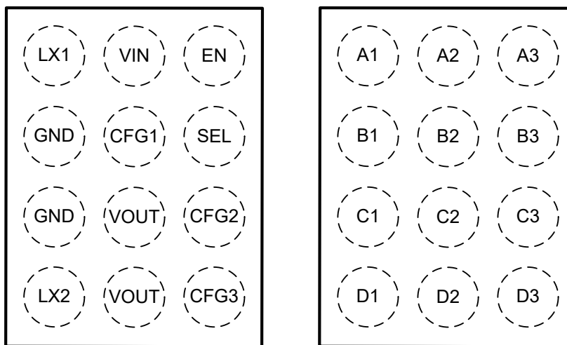
図 4-1. 12-Ball WCSP Package (Top View)
