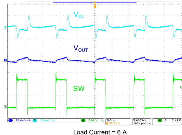
图 9-6. PWM Operation (TPS62A06)
