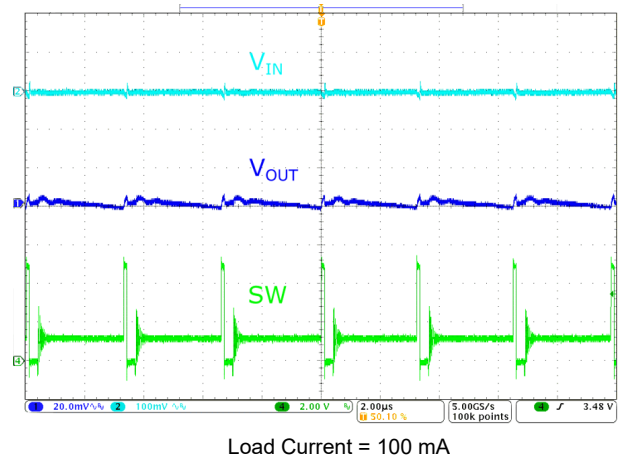
图 9-7. PFM Operation (TPS62A06)
