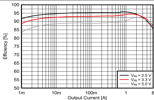
图 9-4. 1.8-V Output Efficiency (TPS62A06)
