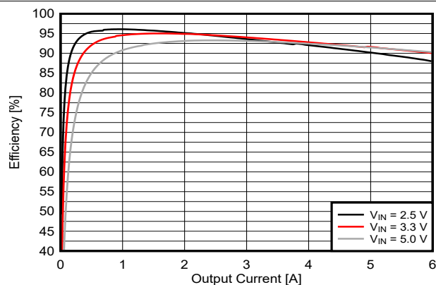
图 9-5. 1.8-V Output Efficiency (TPS62A06A)
