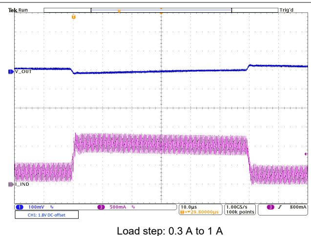
図 8-23. Load Transient
