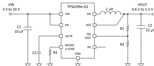
簡略回路図
