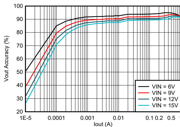
効率と出力電流の関係
