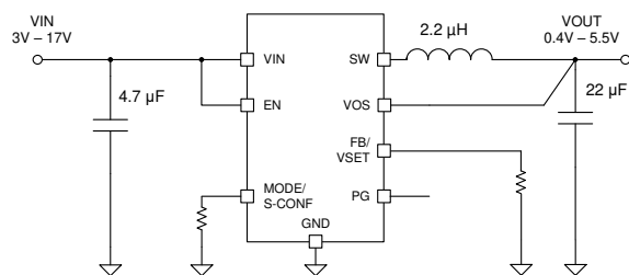
概略回路図
